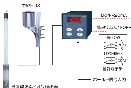
浸漬型塩素イオン検出器
